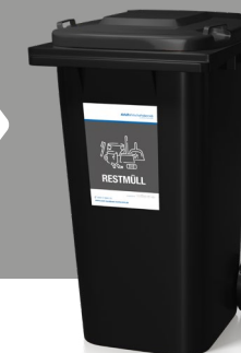
Носовые платки
